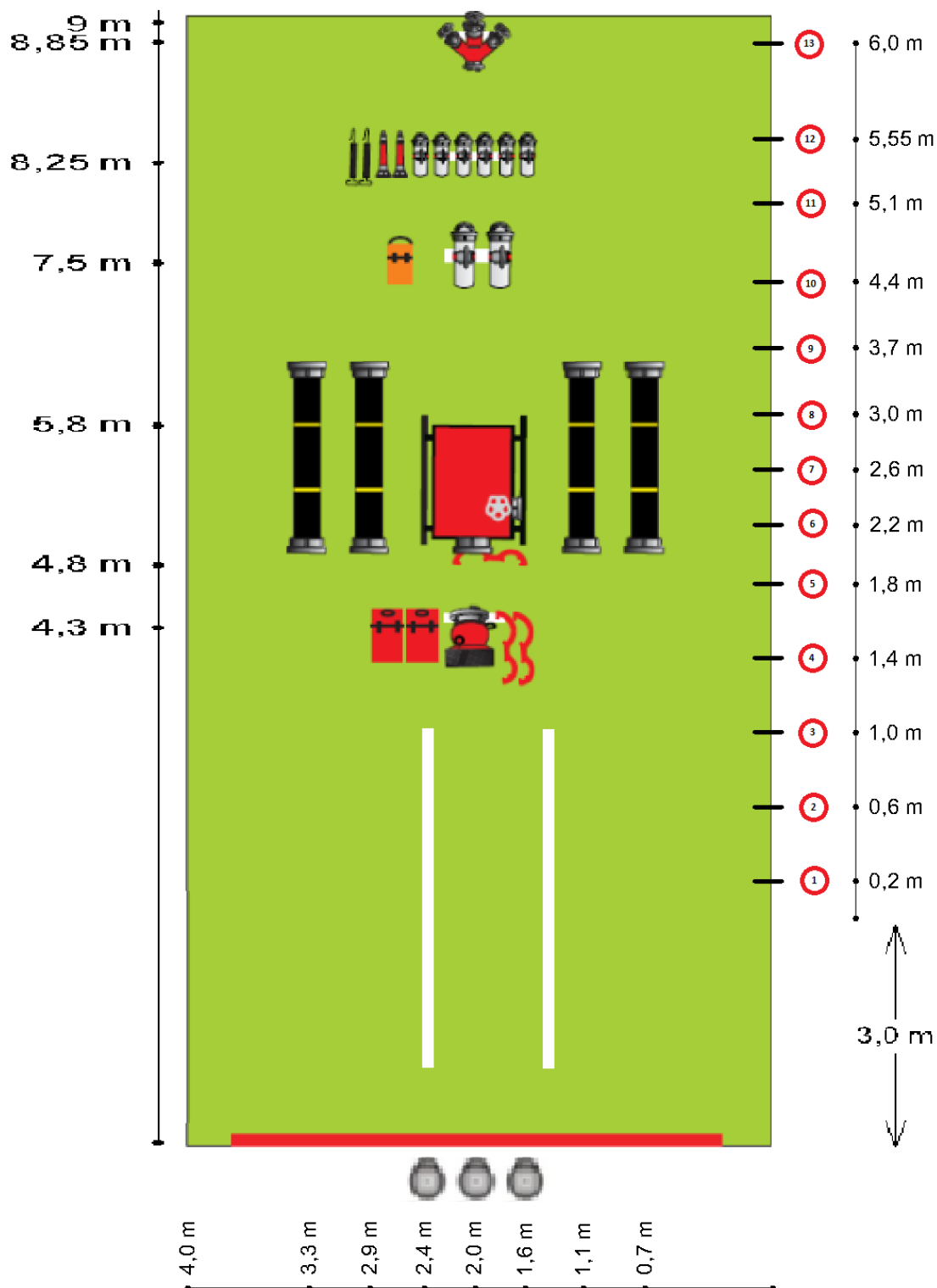
Slika 2: Pravilna postavitvev orodja in opreme pri vaji Postavitvev orodja za vajo z motorno brizgalno
